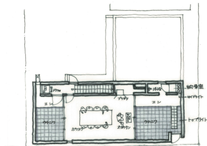
3階平面図
